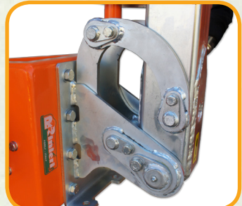
Angolazione barra 215° Tilting cutting bar 215° Angulation barre 215° Drehung Schneidwerk 215° Angulación barra 215°
